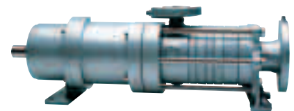
Bomba de canal lateral com transmissão magnética (Modelo SCM)
